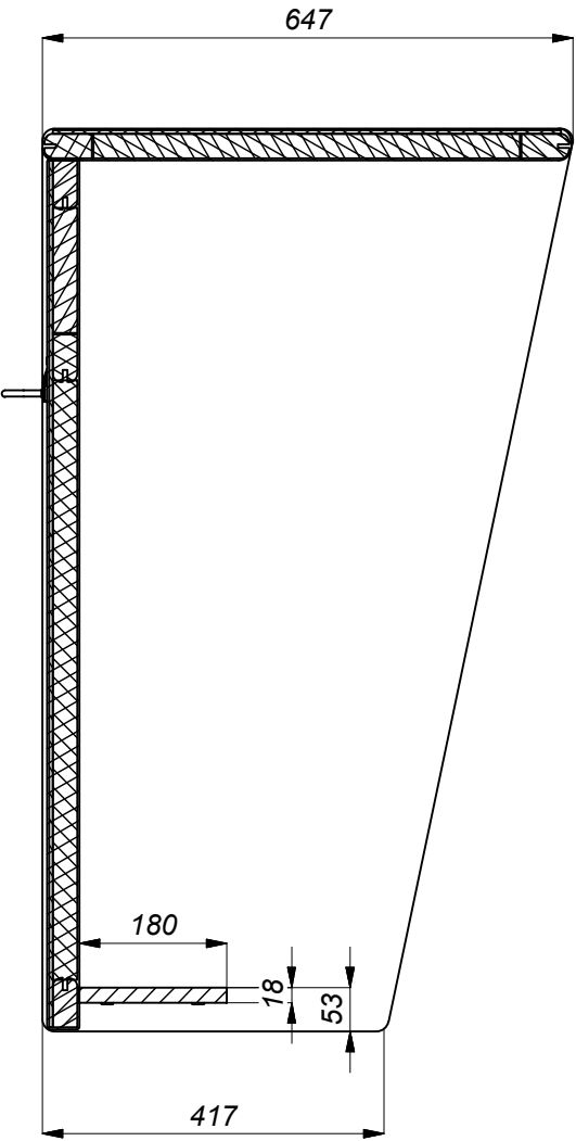
A-A ( 1:10 )
